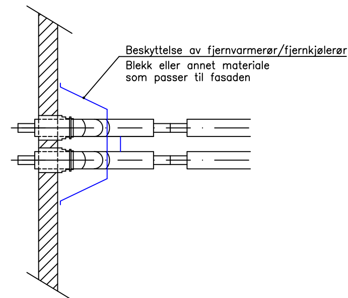
PLAN ALTERNATIV 2 ROM FOR KUNDESENTRAL VED YTTERVEGG
