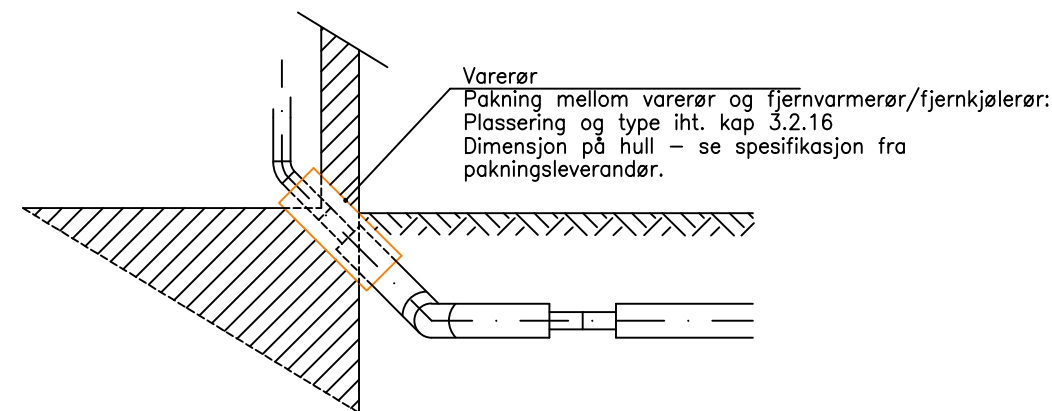
SNITT ALTERNATIV 4 LØSNING 45° INNFØRING
