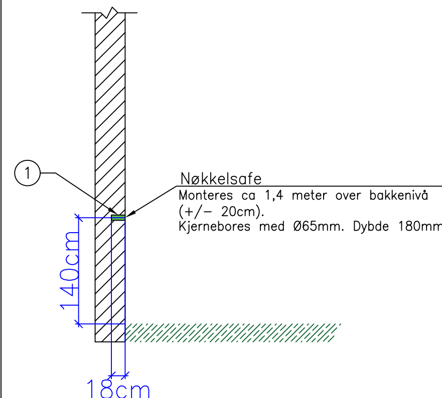
SNITT B
