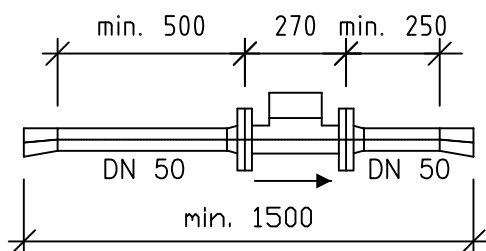
MÅLER DN 50
