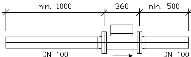
MÅLER DN 100
