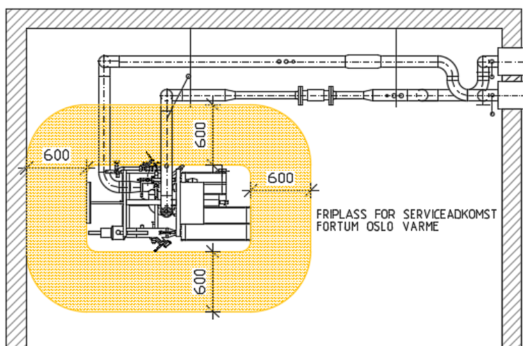
Figur 1: Plassering av kundesentral med serviceadkomst
