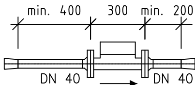
MÅLER DN 40
