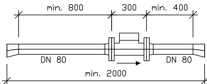
MÅLER DN 80
