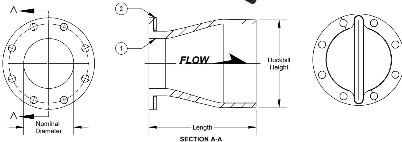
SECTION A-A
