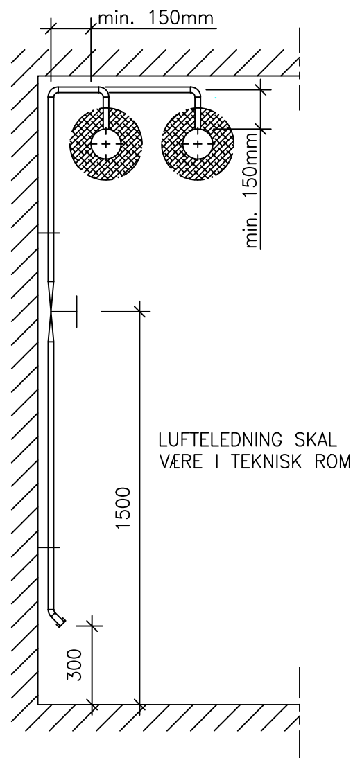
SNITT A-A
