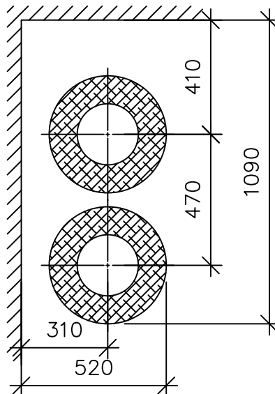
DN80
