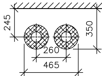
DN80
