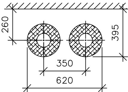
DN100
