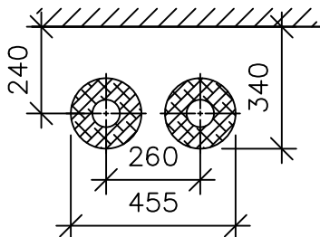
DN65
