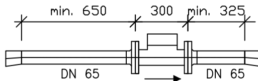
MÅLER DN 65
