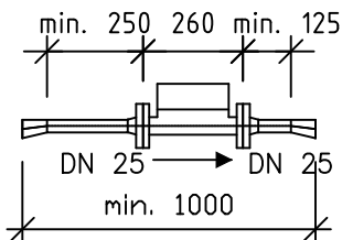
MÅLER DN 25
