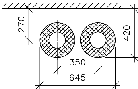
DN125
