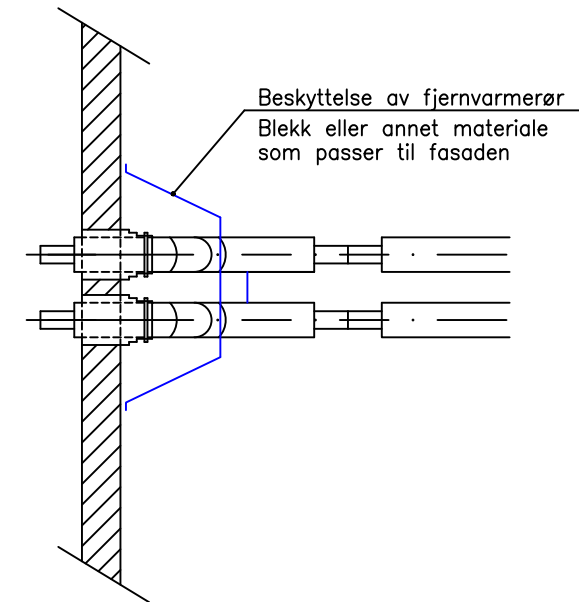
PLAN ALTERNATIV 2 ROM FOR KUNDESENTRAL VED YTTERVEGG
