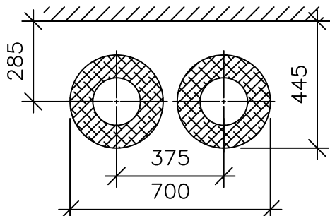
DN150
