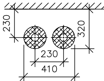
DN50
