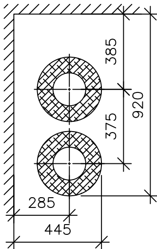
DN65
