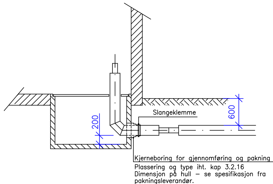
SNITT ALTERNATIV 1 ROM FOR KUNDESENTRAL VED YTTERVEGG
