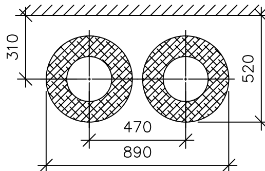
DN200
